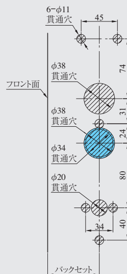
切欠図 (注3)
